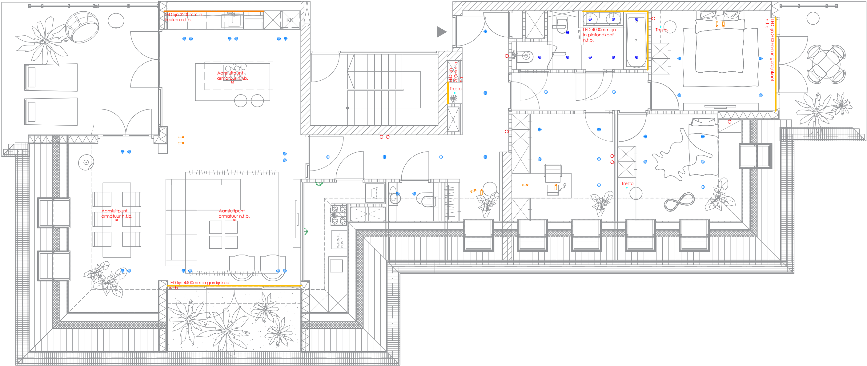
Apartment R16 3e Verdieping
